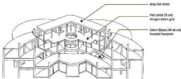
Gambar 9 : Konsep Struktur Bangunan (Penulis, 2023)
